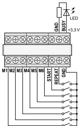
⑤ Conexión para control remoto
