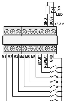
⑤ Branchement pour une gestion à distance
